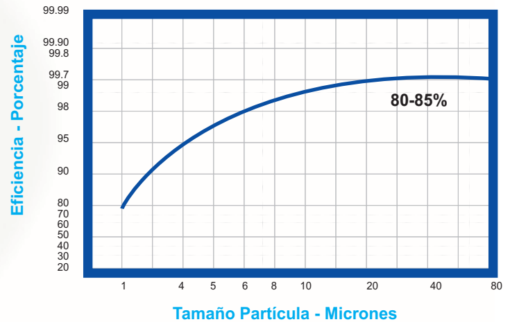
Eficiencia vs. Tamaño Partícula
